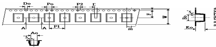
A-A SECTION
